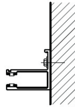
Masonry/Drywall Jamb
